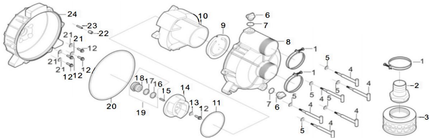
航宇3寸污水泵零部件明细表
